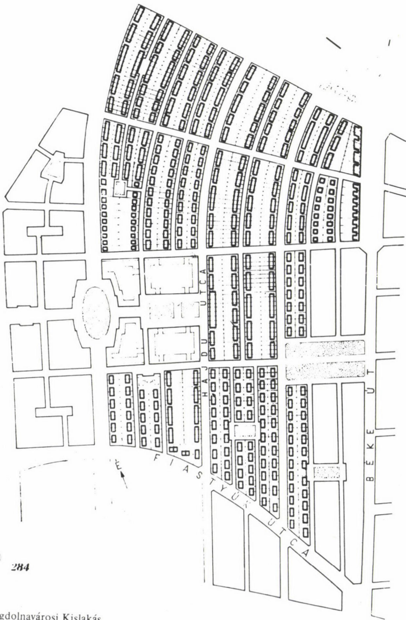
2. Magdolnavárosi Kislakás teleprendezési terve. 1936.
