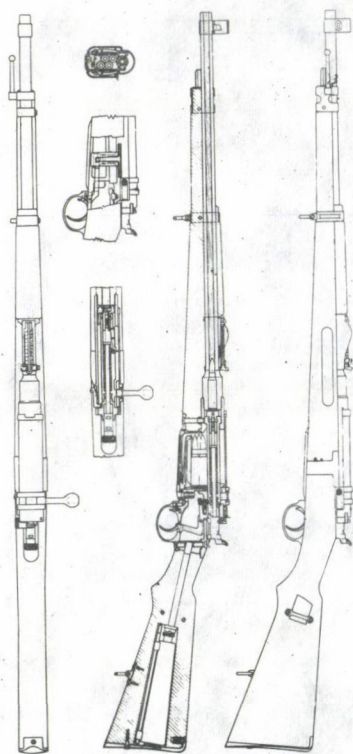
9. 1933 M. kísérleti puská szerkezeti rajzai a Fegyvergyár archív anyagából
