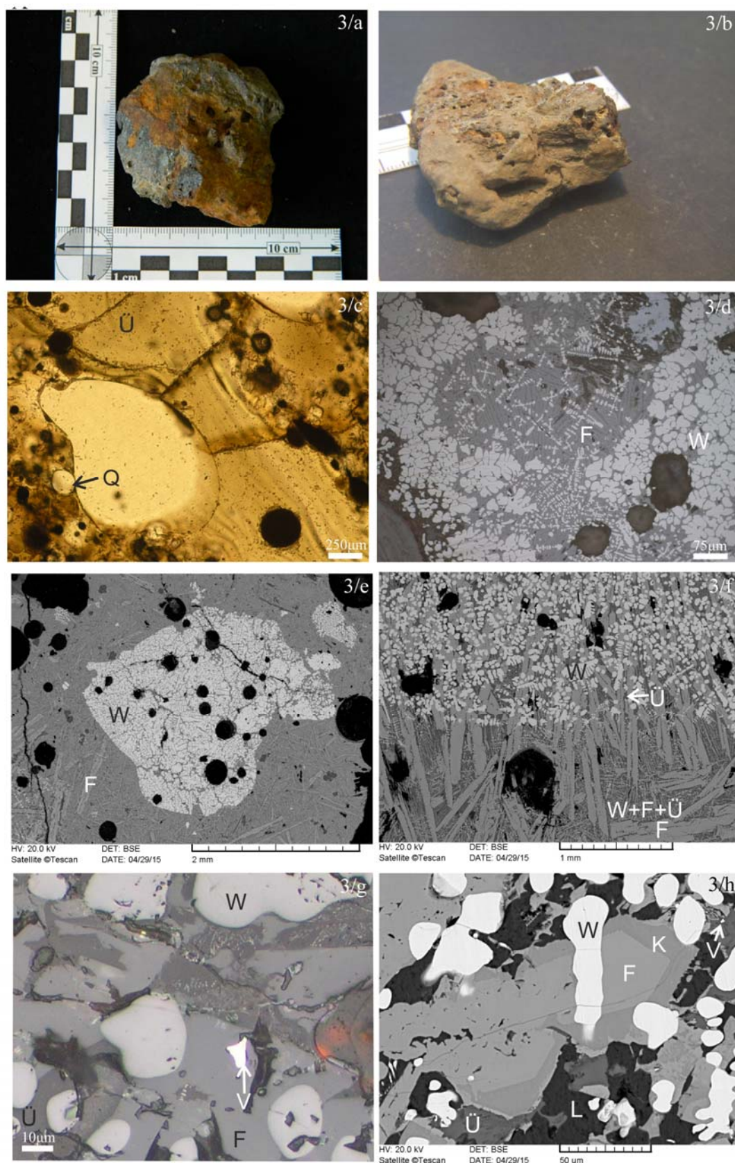
3. ábra: A vizsgált fémsalakok szöveti jellegzetességei makroszkópos, polarizációs mikroszkópos és pásztázó elektronmikroszkópos felvételeken
