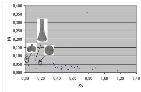
3. ábra: A zalasabari kincs tárgyain végzett elemösszetétel vizsgálat Sb–Ni diagramja; néhány fordított szív alakú csüngő és a négy korongcsüngő, valamint a formaöntött nyersanyagrudként is meghatározható peremes balta adatának kiemelésével
