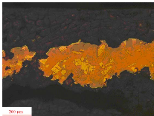
4. ábra: Zalasabari lemezesfejű tű öntést követően megmunkált, hőkezelt szövetszerkezete (optikai mikroszkópos vizsgálat)
